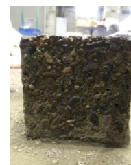
図-2 打継ぎ面
