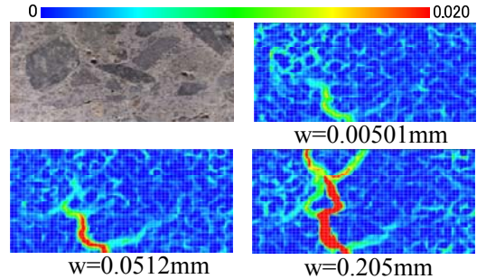
図-3 最大主ひずみ分布 (供試体 3-1-2) 研磨供試体スパン長 160mm
