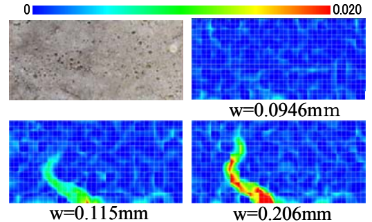
図-2 最大主ひずみ分布 (供試体 3) スパン長 800 mm
