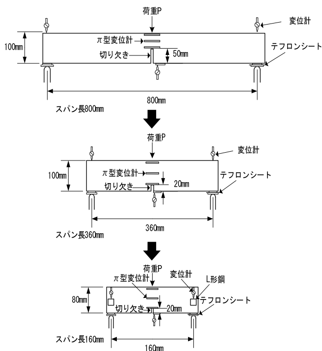
図-1 供試体概要ならびに載荷状況
