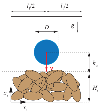
図-2 x_1 - x_3 断面図
