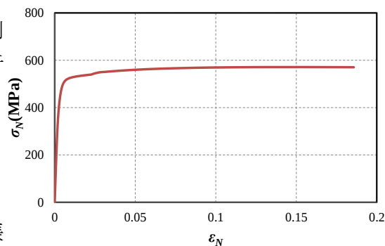
図-1 引張試験結果
