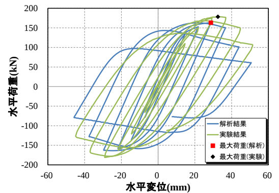
図-4 実験結果と解析結果の比較
