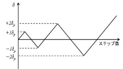
図-2 載荷パターン
