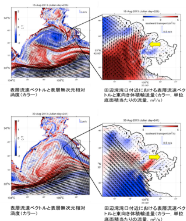
図-3 左: 田辺湾を含む周辺海域における表層無次元相対渦度 (カラー), 右: 東向き体積輸送量。矢印はいずれも表層流速ベクトルである。上: 湾口での流出イベント時, 下: 流入イベント時。
