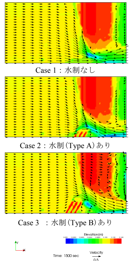
図-6 水制による流れの偏奇と砂州の侵食
