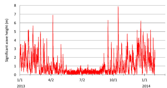
図-3 有義波高(経ヶ岬)
