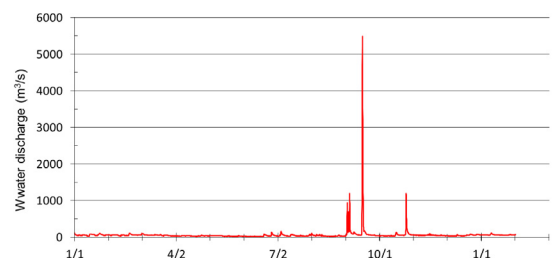
図-4 河川流量(福知山)
