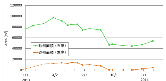
図-2 砂州面積の変化
