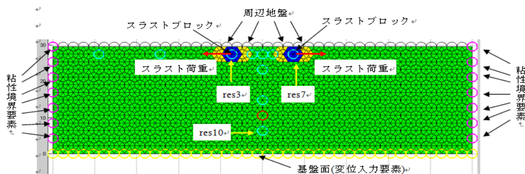
図-2 解析モデル
