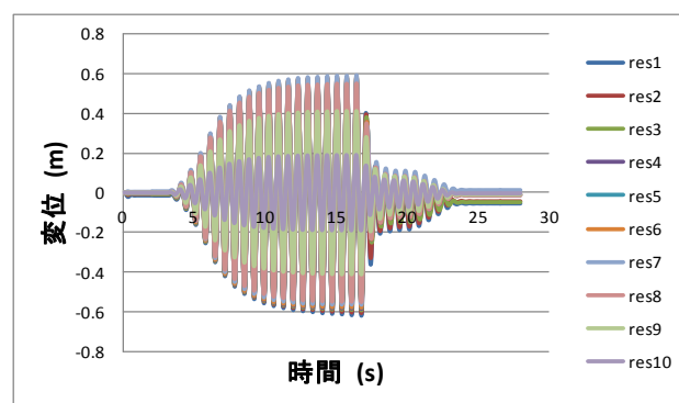
図-6 case1N=3 の観測点の変位波形
