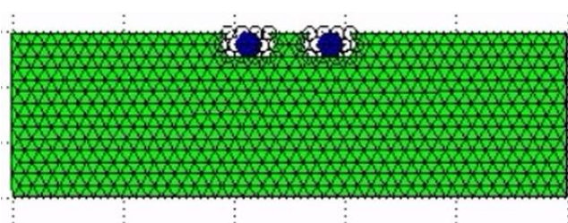
図-5 case1N=3 でのスラストブロック周辺地盤の剥離状況
