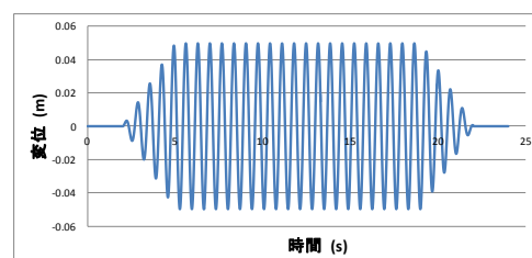
図-1 case1の入力波形
