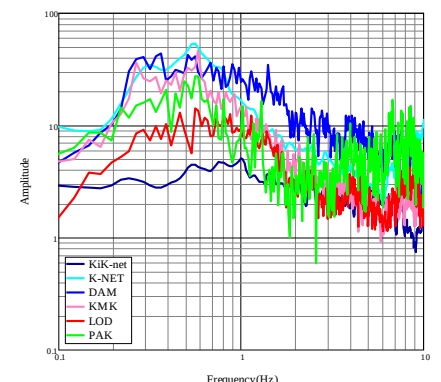
図-3 サイト増幅特性
