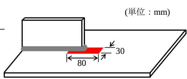
図 4 工法 B
