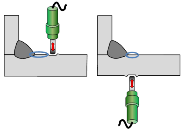
図 2 本研究で検討するピーニング方法
