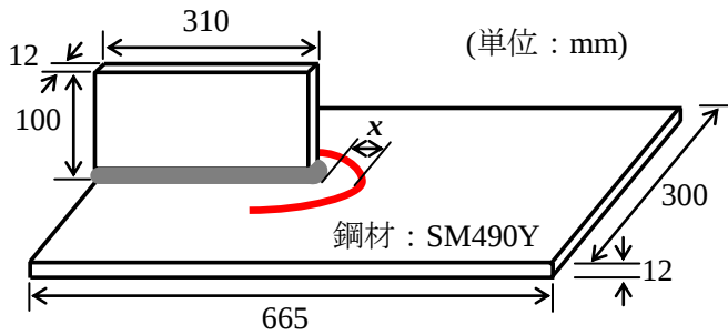
図 3 工法 A
