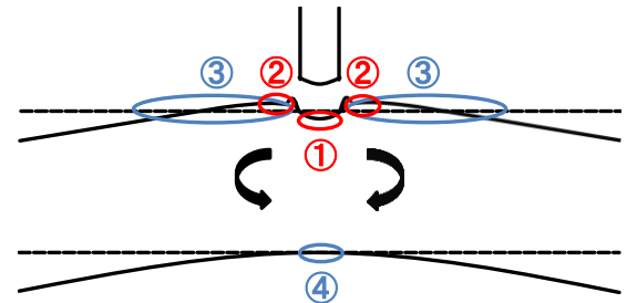
図 1 鋼板の打撃箇所と導入される圧縮応力
