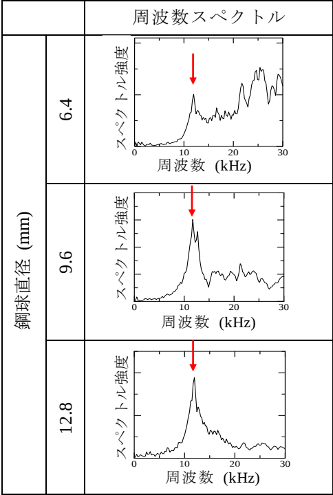
図-4 周波数スペクトル
