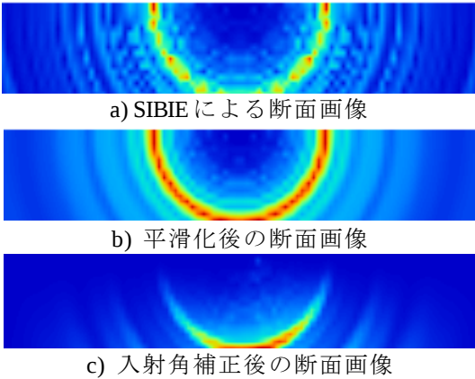
図-3 断面画像の比較
