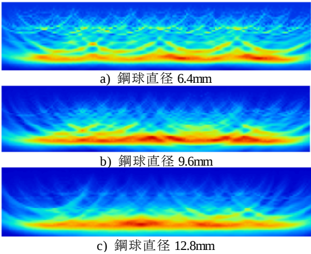
図-5 Accumulated SIBIE による断面画像
