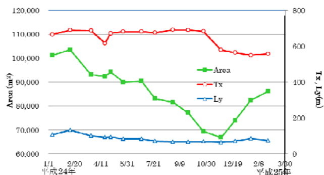
図-2 砂州面積と砂州特性長
