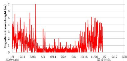
図-4 経ヶ岬における有義波高
