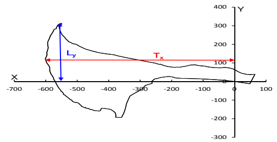
図-5 砂州特性長
