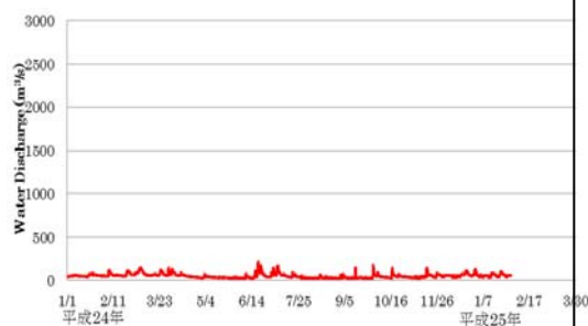
図-3 福知山における河川流量
