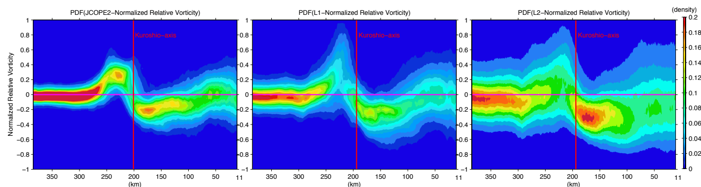
図-3 : JCOPE2, L1, L2 の sub1 の表層無次元相対渦度の PDF
