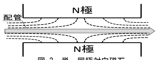
図-3 単一同極対向磁石
