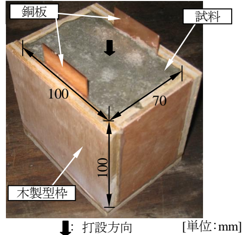
写真-1 型枠および試料の概要
