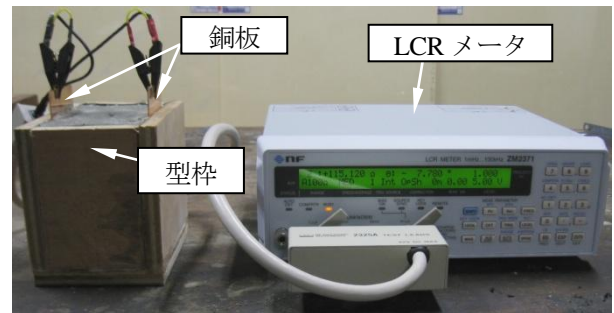
写真-2 計測概要
