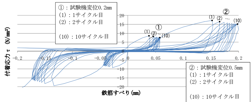
図-3 鉄筋すべり－付着応力関係
