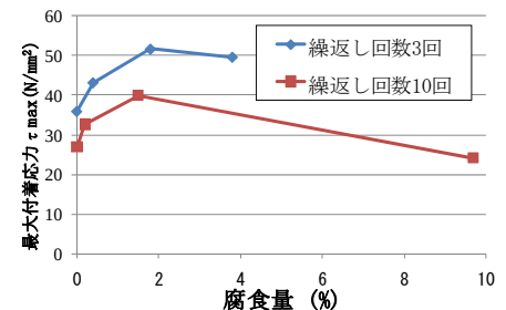
図-4 腐食量－最大付着応力関係
