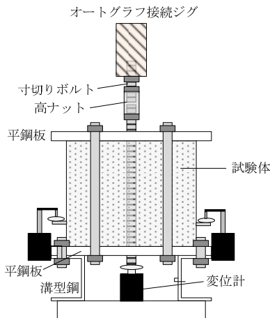
図-2 荷重試験概要図
