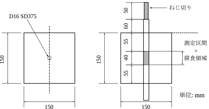
図-1 供試体概要
