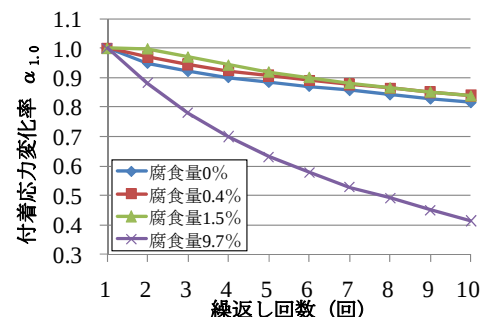
図-5 繰返し回数－付着応力変化率関係
