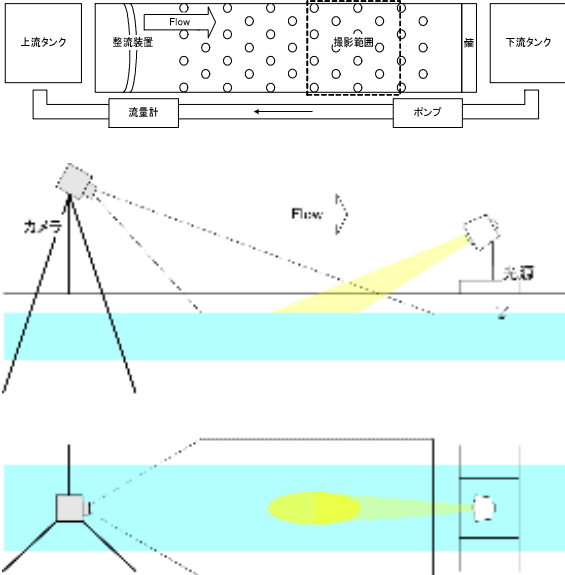
図-1 実験水路
