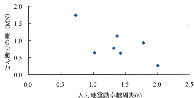
図-4 支承条件の違いによるせん断力の差
