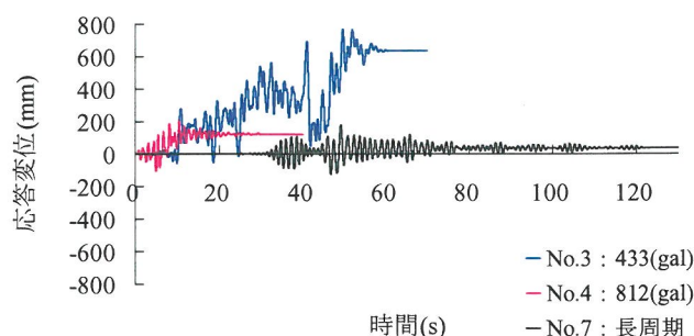
図-2 入力地震動の違いによる時刻歴応答
