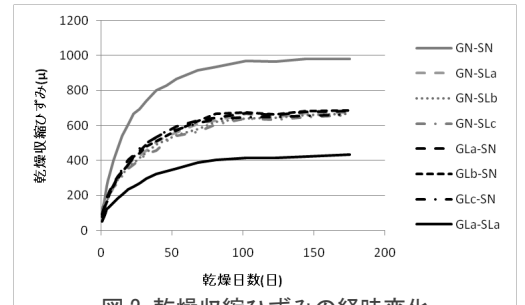
図2 乾燥収縮ひずみの経時変化
