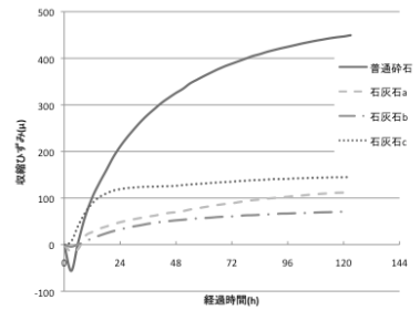
図3 骨材の収縮ひずみの経時変化
