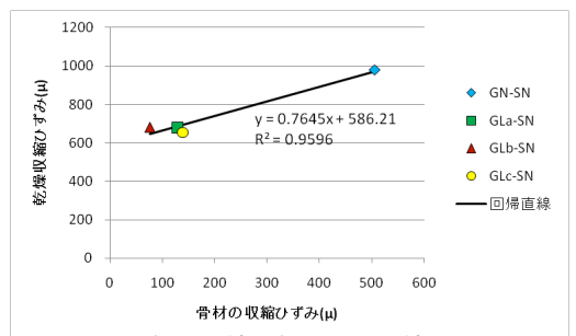
図4 乾燥収縮と粗骨材の収縮の関係
