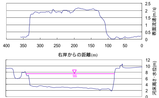
図-4 29.8km における表面流速と河床高さ・水位
