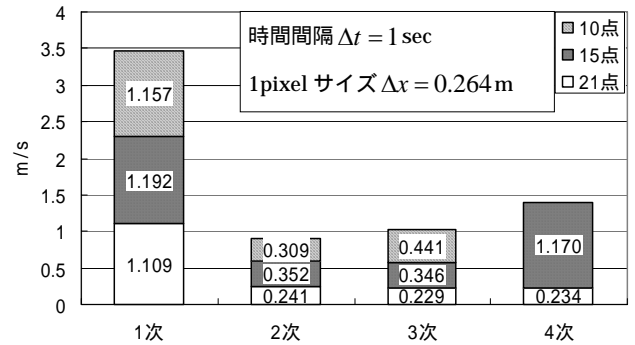
図-1 次数・タイポイント数の違いによる表面流速の rms 値比較
