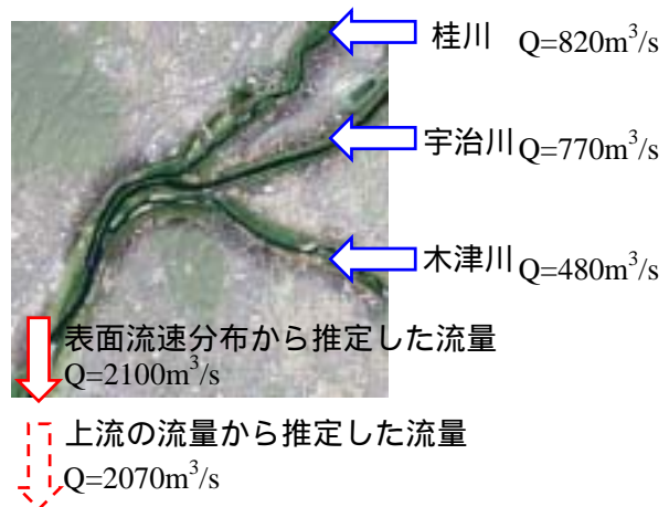
図-5 各河川における流量
