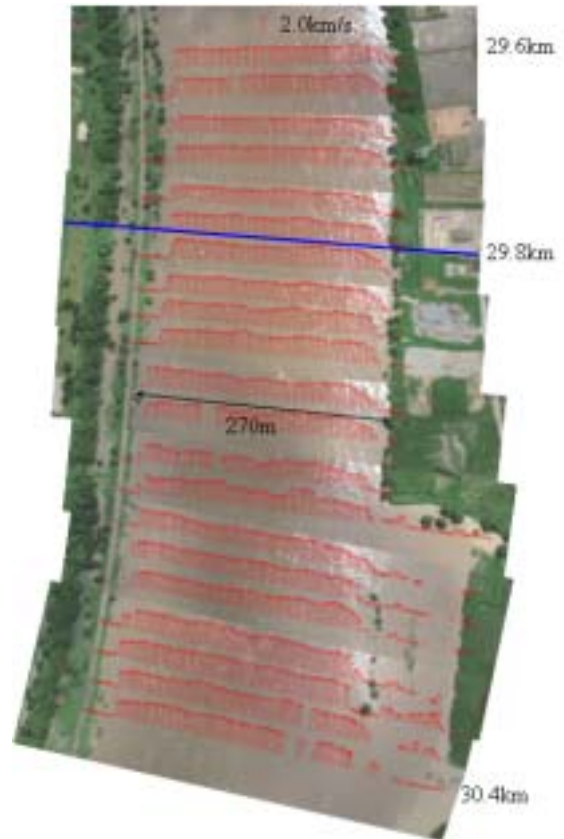
図-3 淀川における表面流速分布
