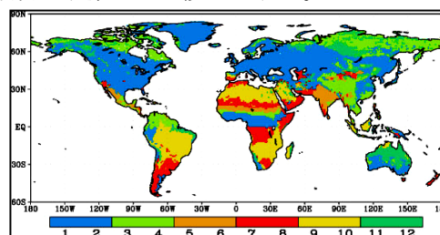
図1 N-NDVIの最小月の分布
