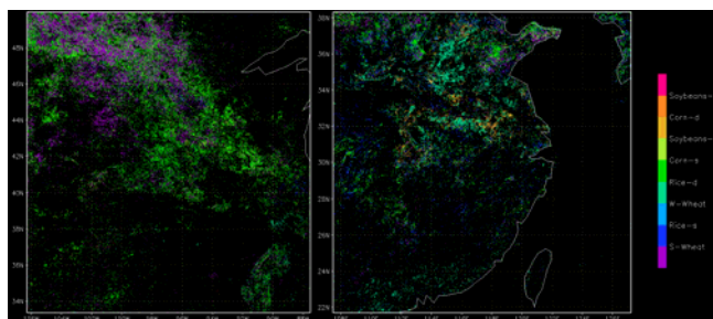
図 2 分類結果(アメリカ五大湖南西部、中国東部)
