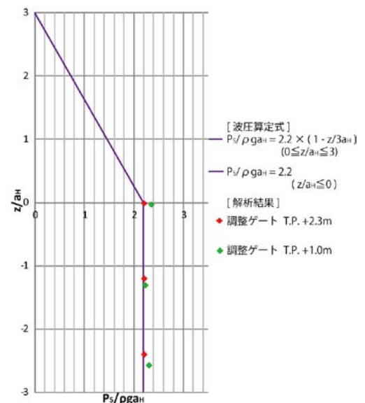
図6 波圧算定式と波圧分布の比較
