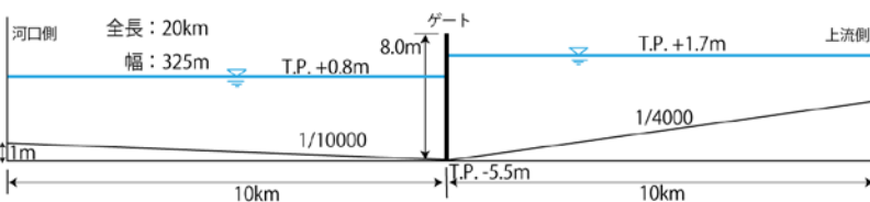
図4 解析地形の概要図
