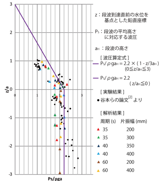
図3 波圧算定式と波圧分布の比較
