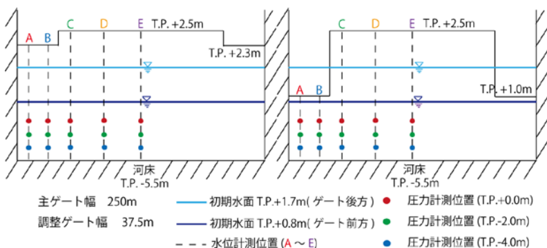
図5 ゲート正面図
