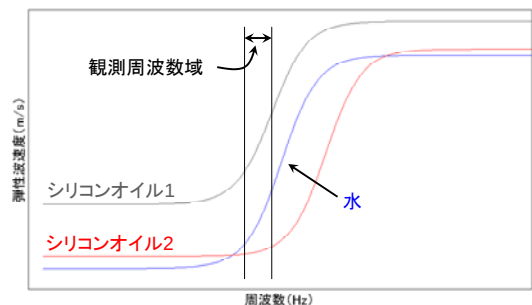
図5 理論曲線と観測周波数域の関係
