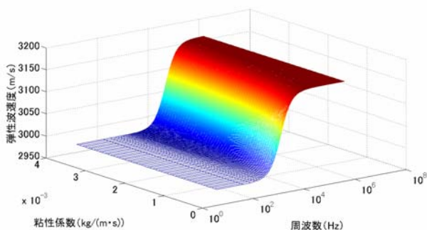
図3 Biot 理論解における粘性係数の影響
