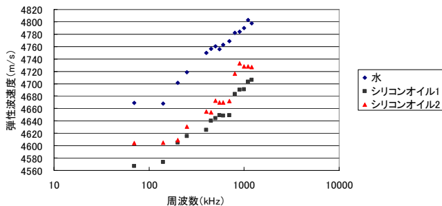
図2 ポーラスストーン 60 測定結果
