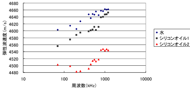
図1 ポーラスストーン 100 測定結果
