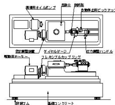
図-1 シェンク式疲労試験機
