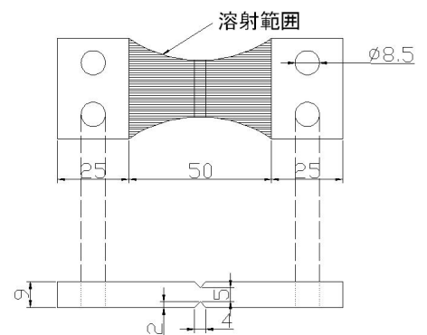
図-2 疲労試験片
