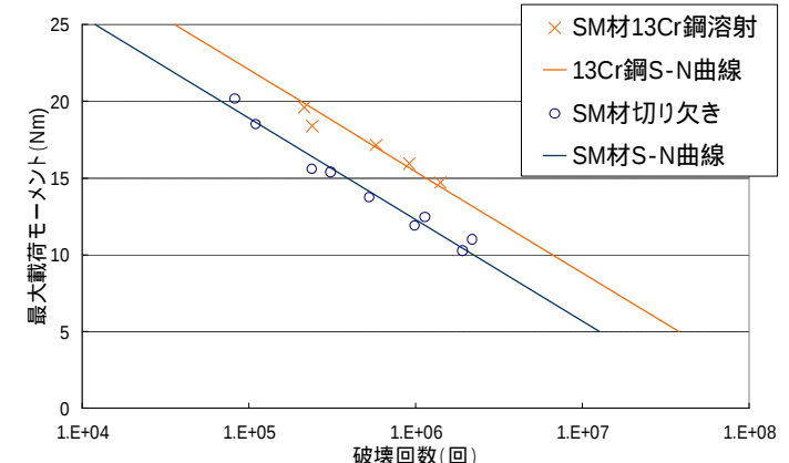
図-5 13Cr 鋼溶射試験片疲労試験結果
