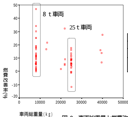
図-2 車両総重量と燃費改善率の関係
