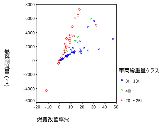
図-3 燃費改善率と燃料削減量の関係
