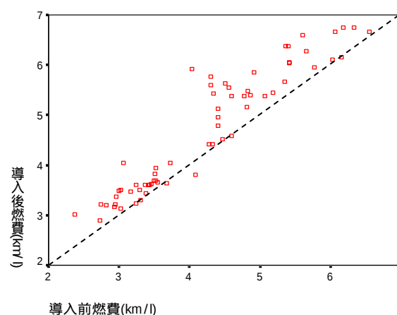
図-1 全車両の導入前燃費と導入後燃費の関係
