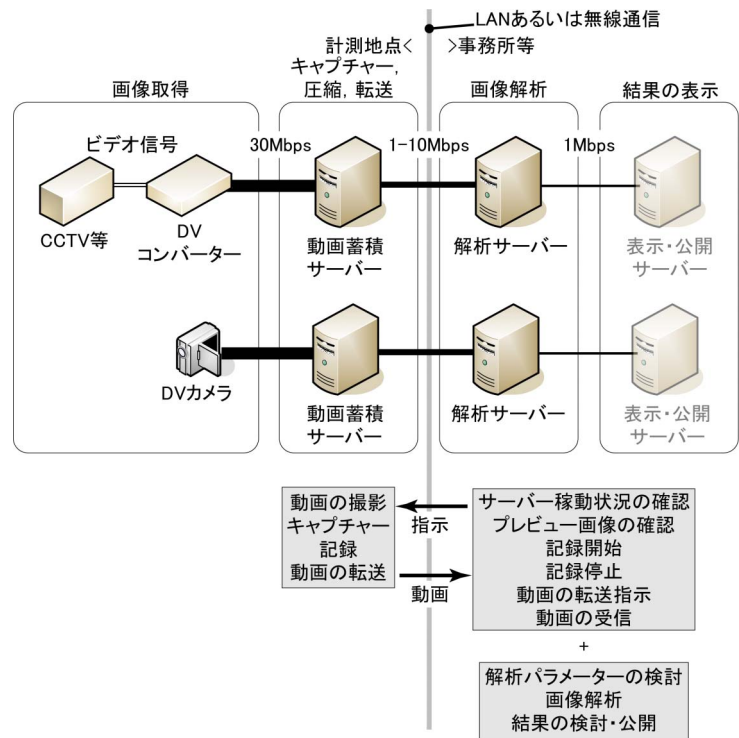
図1 機器および機能分担の構成
