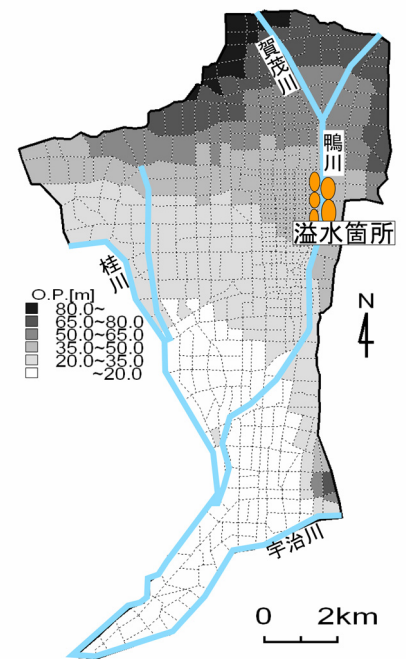
図-2 地盤高&amp;溢水箇所図
