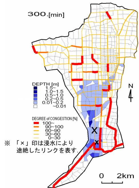
図-6 浸水時解析結果
