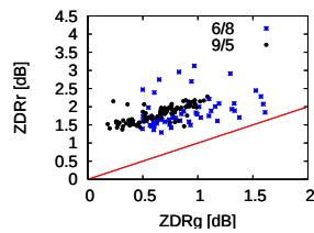
図2 観測された Z_{DR} の観測精度
