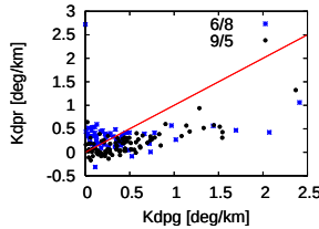
図3 観測された K_{DP} の観測精度
