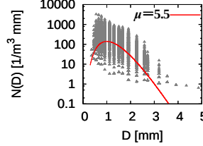
図4 9/5 0:00~8:00の粒径分布
