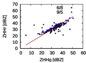
図1 観測された Z_{HH} の観測精度
