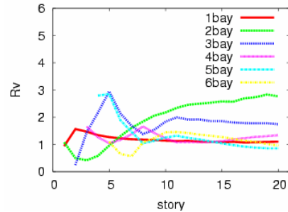
図 4： 倒壊エネルギーの比較
