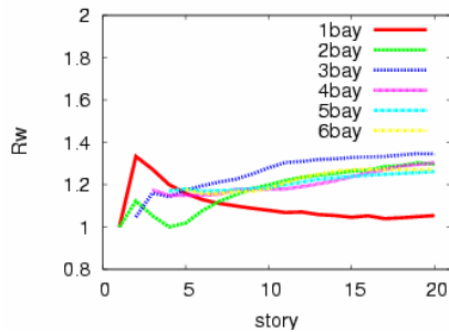
図 3： 倒壊荷重の比較
