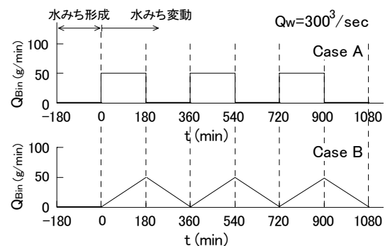
図-1 給砂条件
