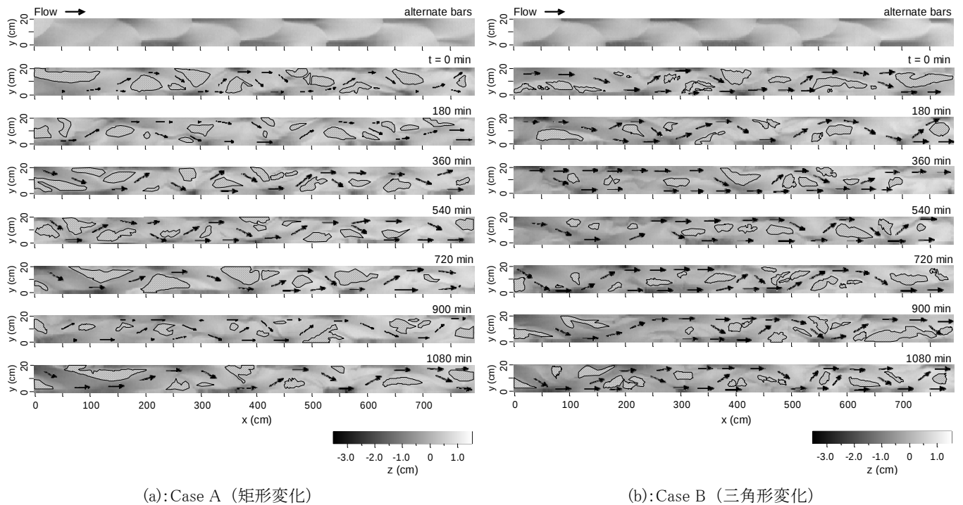
図-3 河床形状と流砂方向の時間変化
