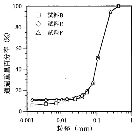
図-1 試料の粒径加積曲線
