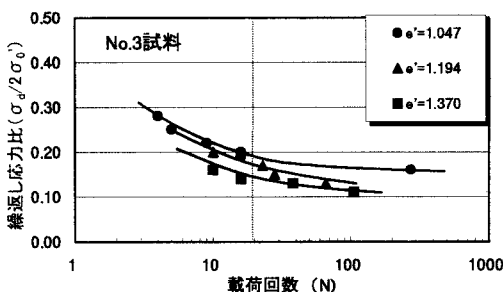
図-4 繰返し応力比と載荷回数の関係
