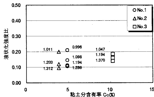
図-6 液状化強度比と粘土分含有率の関係
