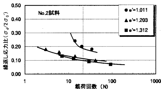
図-3 繰返し応力比と載荷回数の関係
