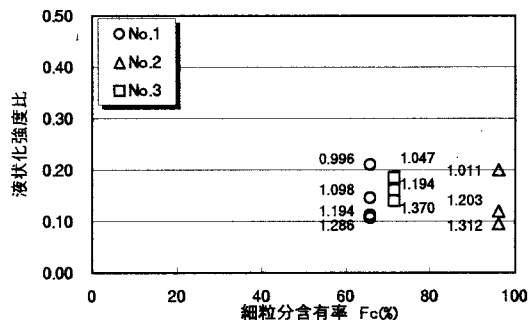
図-5 液状化強度比と細粒分含有率の関係
