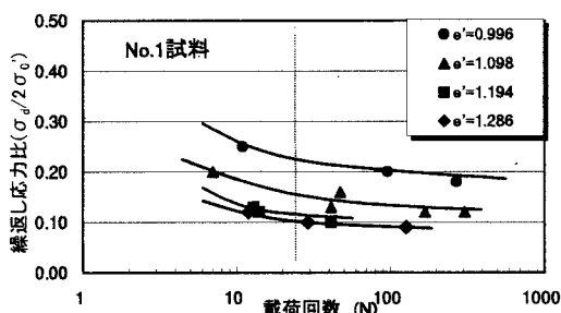
図-2 繰返し応力比と載荷回数の関係
