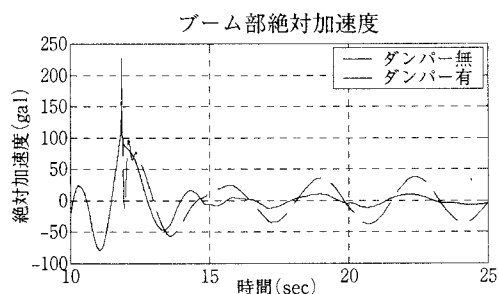
図7 ダンパーの付加による応答比較
