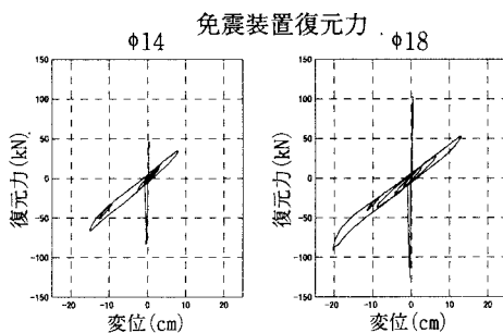
図5 ハイブリッド実験結果
