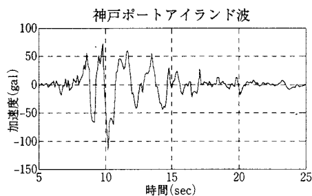
図4 入力地震動 (1/3 スケール)
