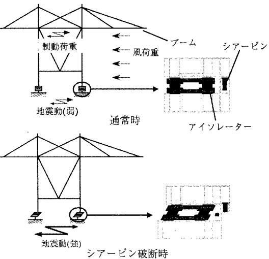
図1 シアーピン付免震装置
