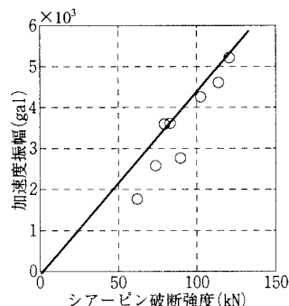
図6 シアーピン破断強度と破断時高次モードにおける免震装置加速度振幅との関係
