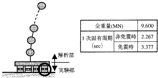
図3 簡易動的モデル
