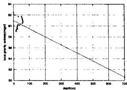
図1: 局所的重力異常と基盤深度との関係
