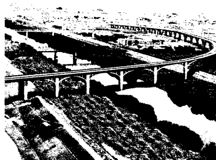
写真-1 アーチ系の桁橋 (逆ランガー連続桁橋)
