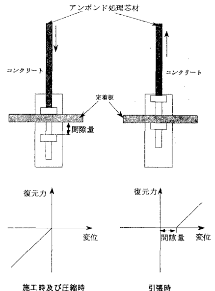
図3 間隙付き定着の模式図
