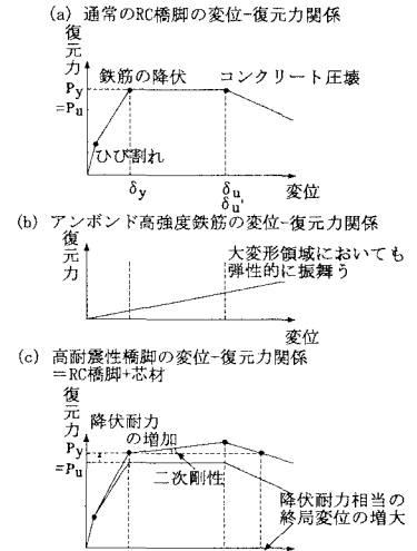
図2 アンボンド化した芯材を挿入する効果
