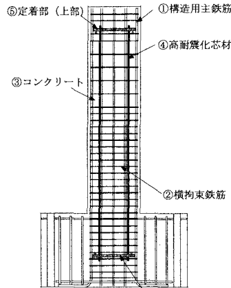
図1 高耐震化芯材を用いたRC橋脚の模式図
