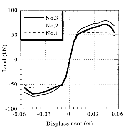
図 5 スケルトン曲線
