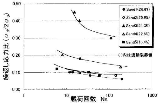
図-4 液状化強度曲線
