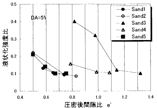
図-5 液状化強度比と圧密後間隙比の関係
