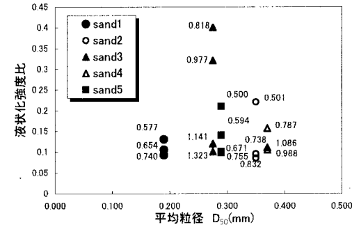
図-2 平均粒径と液状化強度比の関係
