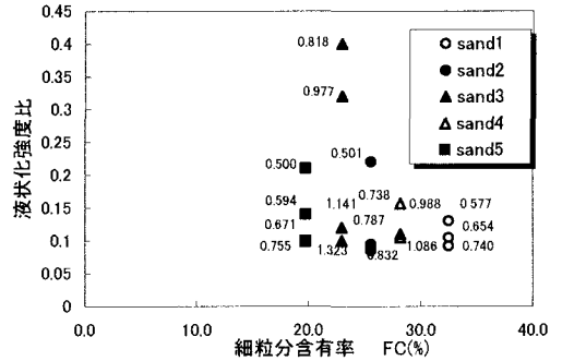
図-3 細粒分含有率と液状化強度比の関係
