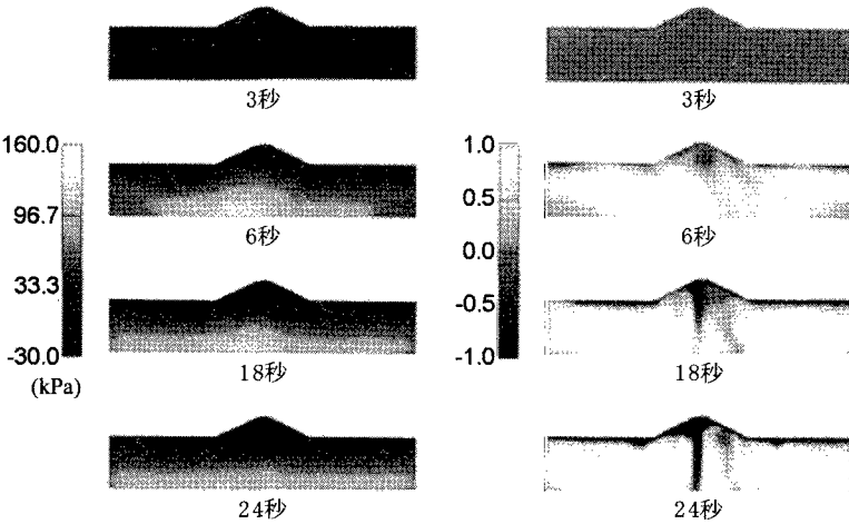
図 5：間隙水圧分布
