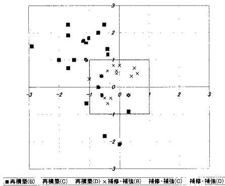
図 3 RC 構造橋脚における橋脚移動量 (°)
