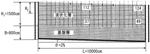
図-2 地盤モデル
