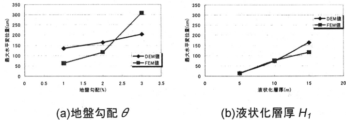
図-5 各要因と側方流動量の関係
