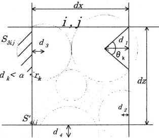
図-1 メッシュの間隙面積
