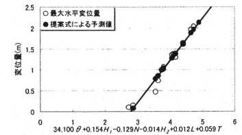
図-6 解析結果と予測値の分布
