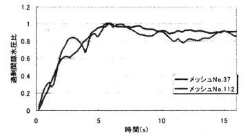
図-4 過剰間隙水圧比
