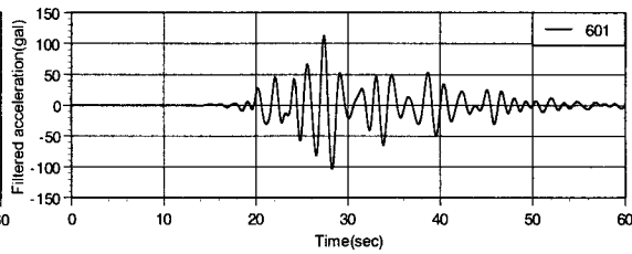
(3) 今回手法によるフィルタ波（次数 601，カイザー窓）
