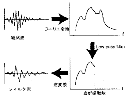
図-1 フィルタ波の算定
