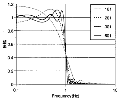
図-2 フィルタ特性(次数による)
