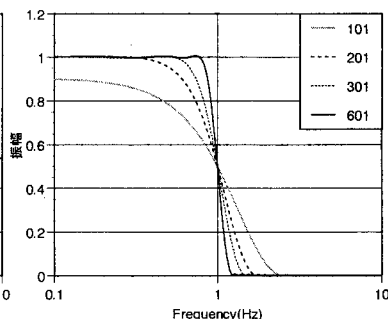
図-4 フィルタ特性(カイザー窓)
