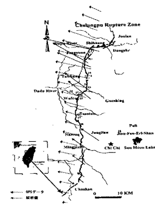
図-4 台湾集集地震におけるGPSデータと解析値の比較(水平変位、修正後)
