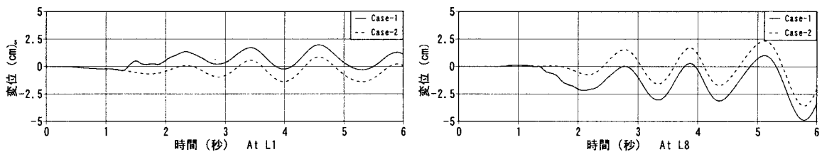
図 5. Case-1 と Case-2 の変位応答の比較
