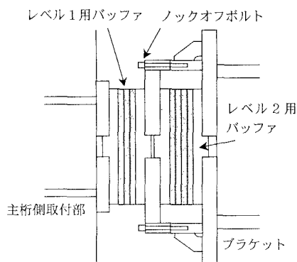
図-2 マルチレベルバフファの平面図
