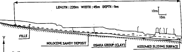
図-1 解析対象斜面
