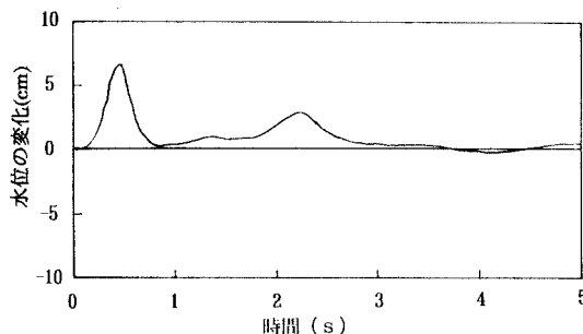
図-2 水位の変化 (汀線より 3m)
