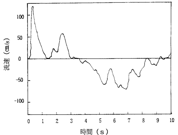
図-4 流速の変化(汀線より1m)
