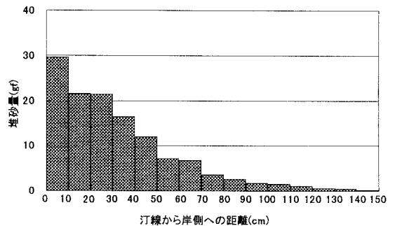
図-5 堆砂量の距離的变化
