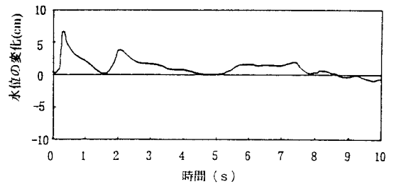
図-3 水位の変化(汀線より1m)
