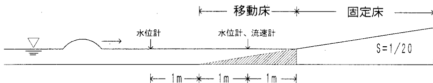
図-1 実験水槽
