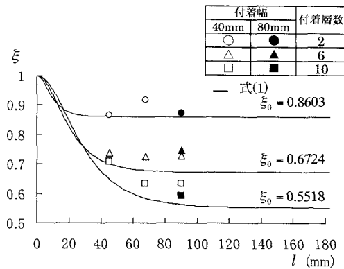
図-4 \xi と l の関係
