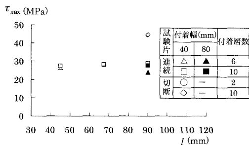
図-6 \tau_{\max} と l の関係
