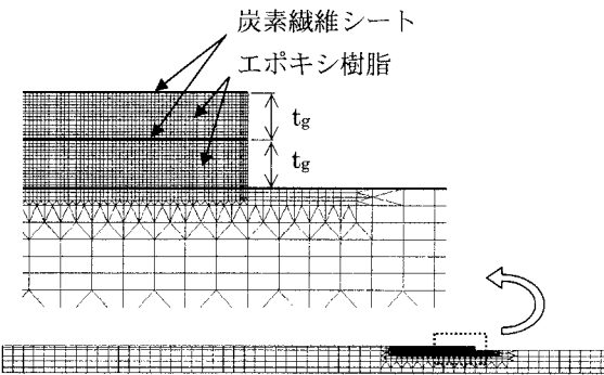
図-2 要素分割〔連続〕
