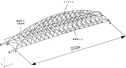
図-1 西宮港大橋の置換骨組構造モデル
