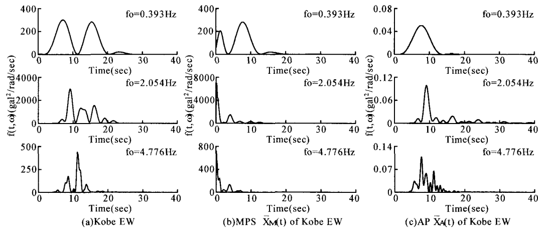
図-3 Kobe EW の非定常スペクトル; 同記録の MPS の非定常スペクトル; 同記録の AP の非定常スペクトル (fo=0.393Hz, 2.054Hz と 4.776Hz)
