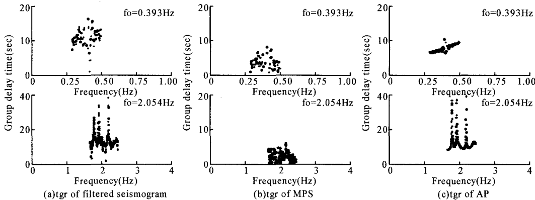
図-2 Kobe EW の帯域波と同帯域波の MPS, AP の群遅延時間(fo=0.393Hz と 2.054Hz)
