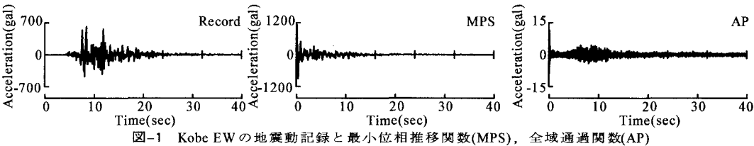
図-1 Kobe EW の地震動記録と最小位相推移関数(MPS), 全域通過関数(AP)
