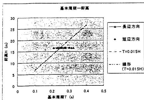
図 3 基本周期—軒高
