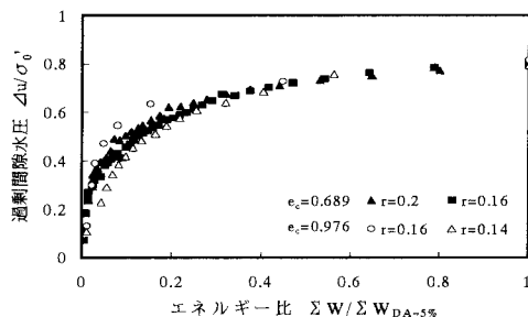
図-4 過剰間隙水圧比とエネルギー比の関係(TB)
