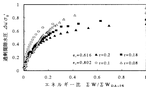
図-5 過剰間隙水圧比とエネルギー比の関係(RB)
